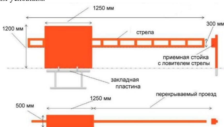
Рисунок 1 – Внешний вид и приблизительные габариты ОУ
