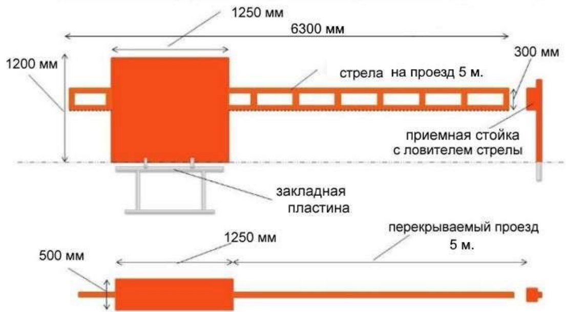
Рис. 2. Габаритные размеры
