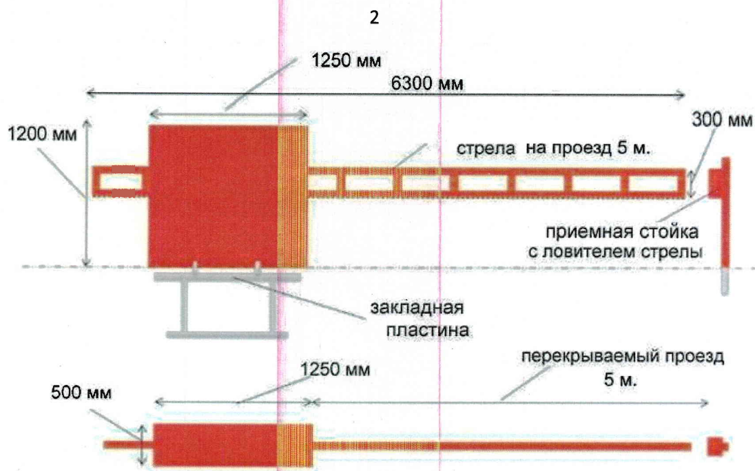
Рис. 2. Габаритные размеры
